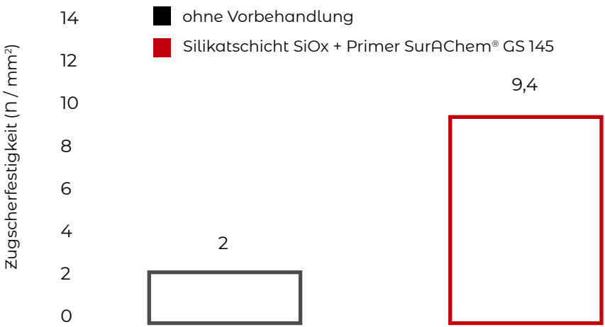
Grafik 1: Zugscherfestigkeitstest mit dem Haftpromotor SurAChem® GS 145 auf PMMA Material
