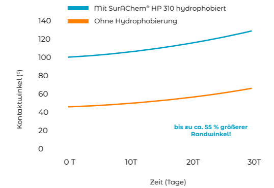
Graphik 1b: Kontaktwinkelmessungen auf Keramikoberfläche mit und ohne Anwendung des Hydrophobierers SurAChem® HP 310
