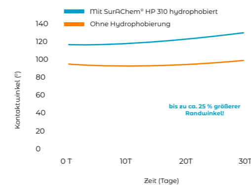
Graphik 1c: Kontaktwinkelmessungen auf Kunststoffoberfläche (PVC) mit und ohne Anwendung des Hydrophobierers SurAChem® HP 310
