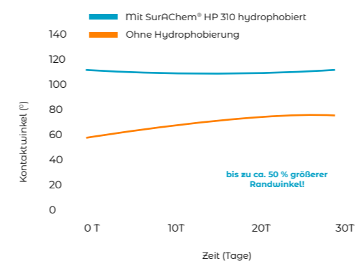
Graphik 1a: Kontaktwinkelmessungen auf Glasoberfläche mit und ohne Anwendung des Hydrophobierers SurAChem® HP 310
