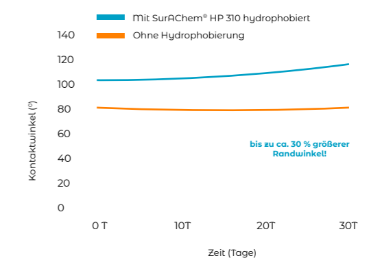
Graphik 1d: Kontaktwinkelmessungen auf Metalloberfläche (Aluminium) mit und ohne Anwendung des Hydrophobierers SurAChem® HP 310
