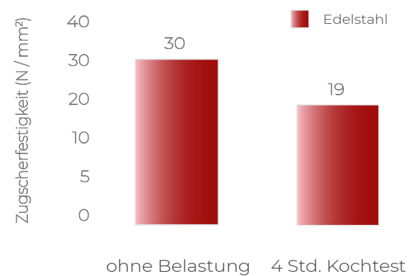
Grafik 1: Zugscherfestigkeitstests mit dem Klebstoff SurABond® SK 250 S
