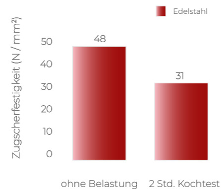
Grafik 1: Zugscherfestigkeitstests mit dem Klebstoff SurABond® SK 231-1.
