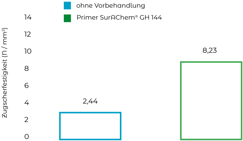
Grafik 1: Zugscherfestigkeitstest mit dem Haftpromotor SurAChem® GH 144 auf Glasmaterial
