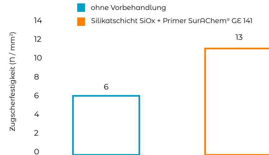
Grafik 1: Zugscherfestigkeitstest mit dem Haftpromotor SurAChem® GE 141 auf PPS / Edelstahl sandgestrahlt
