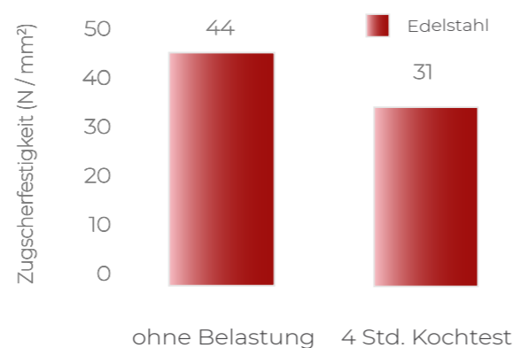
Grafik 1: Zugscherfestigkeitstests mit dem Klebstoff SurABond® SK 310
