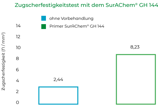
Grafik 4: Zugscherfestigkeitstest mit dem Haftpromotor SurAChem® GH 144 auf Glasmaterial
