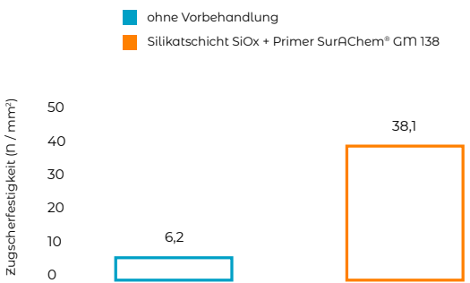
Grafik 1: Zugscherfestigkeitstest mit dem Haftpromotor SurAChem® GM 138 auf Glas / Edelstahl sandgestrahlt
