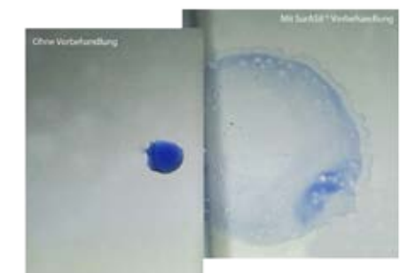
Bild 2: Effekt der Oberflächensilikatisierung auf Aluminium-Material.
