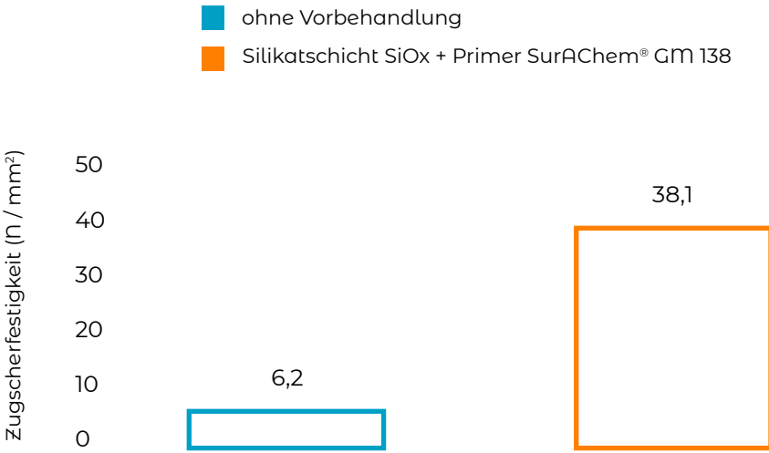
Grafik 1: Zugscherfestigkeitstest mit dem Haftpromotor SurAChem® GM 138 auf Glas / Edelstahl sandgestrahlt
