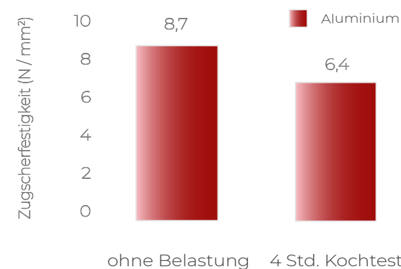
Grafik 1: Zugscherfestigkeitstests mit dem Klebstoff SurABond® SK 289
