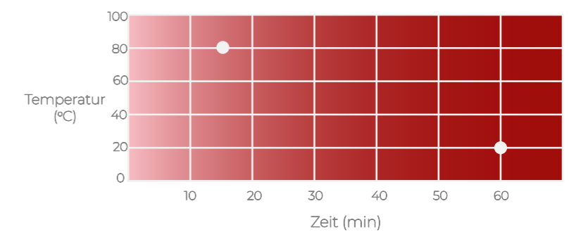
Ablösbarkeit mit dem Deblocker SurABond® HR 90
