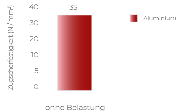
Grafik 1: Zugscherfestigkeitstests mit dem Klebstoff SurABond® HS 24
